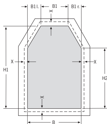
VS 6 Šešiakampis
